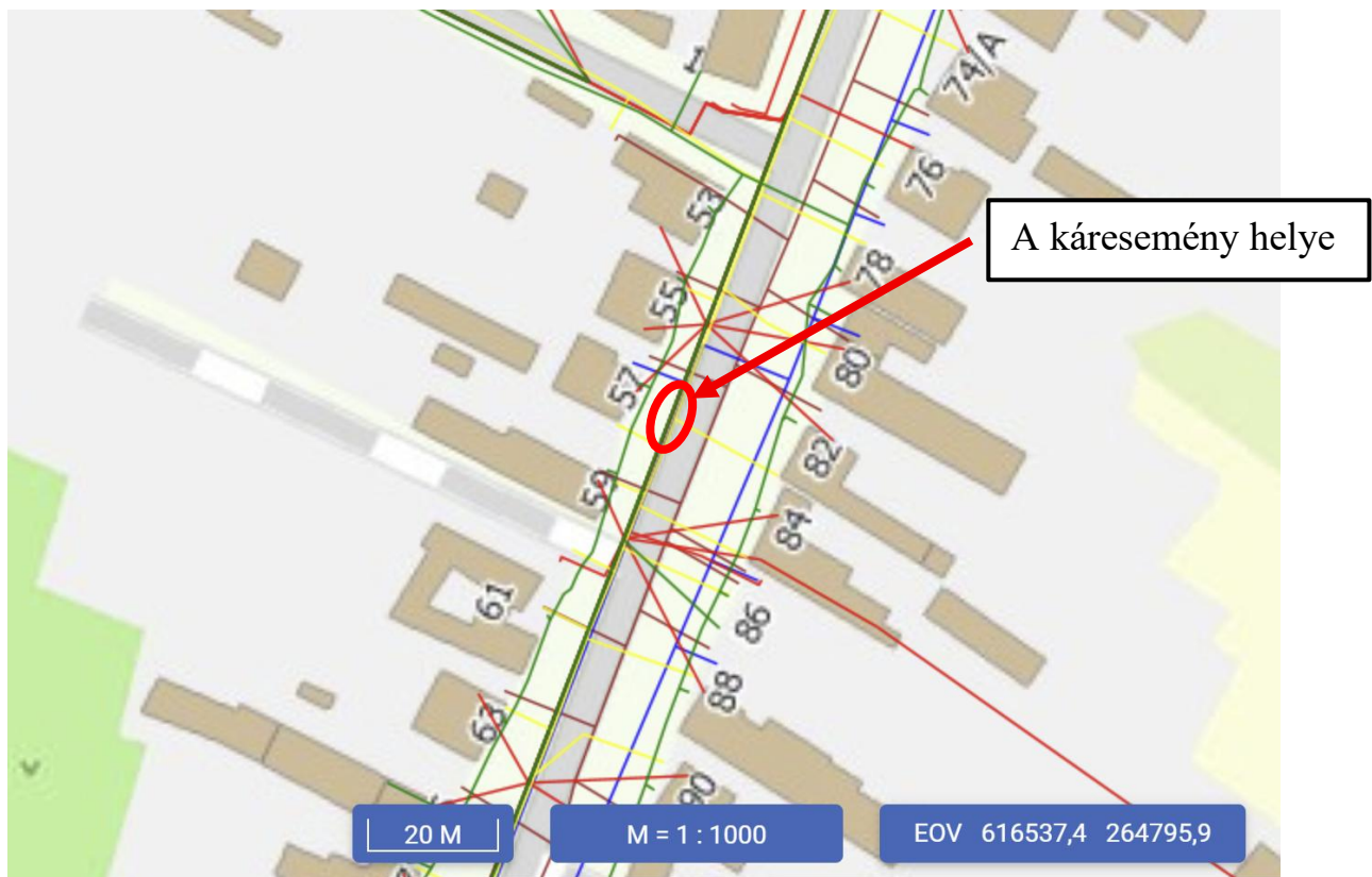
1. ábra - közműtérkép
